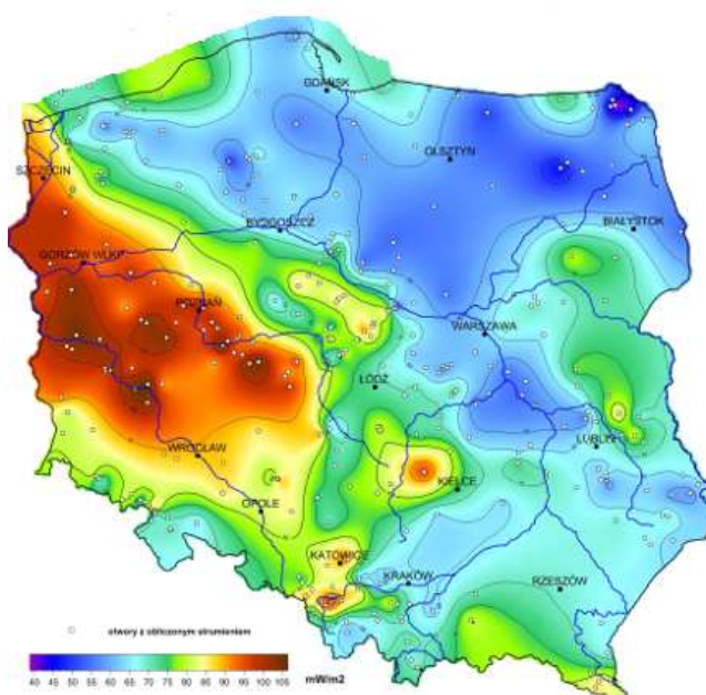
Rysunek nr 39. Mapa gęstości ziemskiego strumienia ciepłego dla obszaru Polski
